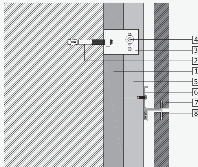
SECCIÓN VERTICAL
