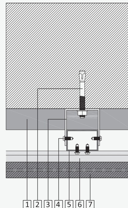
SECCIÓN HORIZONTAL
